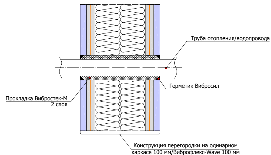
8.3.2 Схема пропуска труб отопления/водопровода через конструкцию перегородки на одинарном каркасе 100 мм/Виброфлекс-Wave 100 мм
