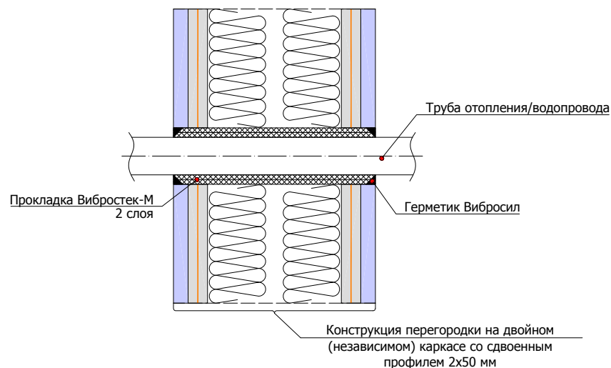
8.3.3 Схема пропуска труб отопления/водопровода через конструкцию перегородки на двойном (независимом) каркасе со сдвоенным профилем 2x50 мм
