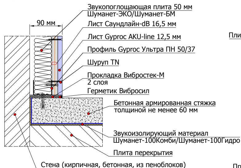
4.1.1 Примыкание облицовки стены на независимом каркасе 50 мм к конструкции "плавающего" пола
