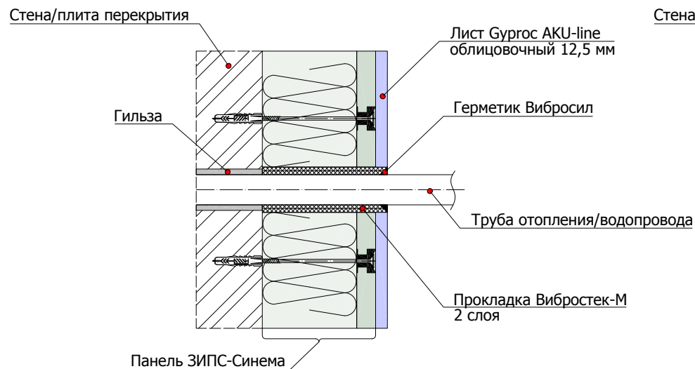
8.4.3 Схема пропуска труб отопления/водопровода через конструкцию панельной системы ЗИПС-Синема
