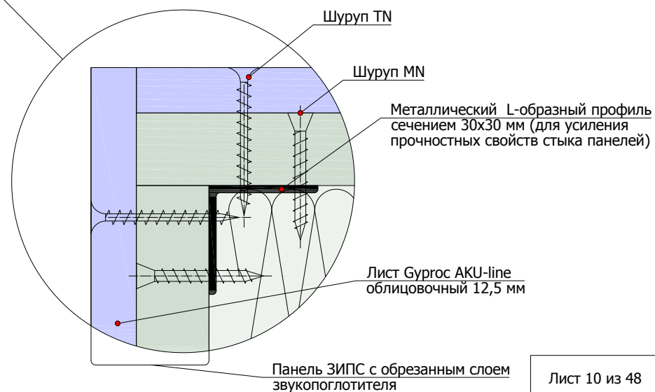
2.1.5 Узлы крепления панелей ЗИПС при монтаже внешнего угла
