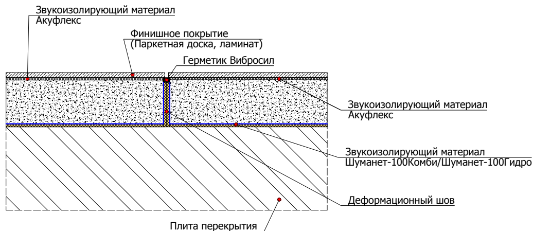
6.1.3 Схема применения материала Акуфлекс под финишным покрытием в сочетании с конструкцией плавающего пола с применением звукоизолирующего материала Шумостоп-К2 в 2 слоя
