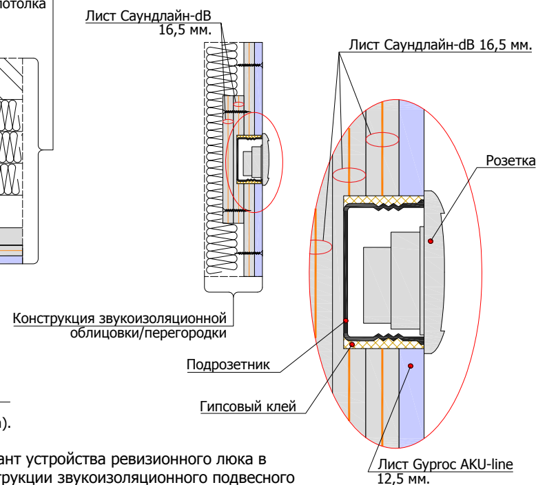
8.2.1 Схема устройства встроенных розеток в конструкциях звукоизоляционных облицовок и перегородок
