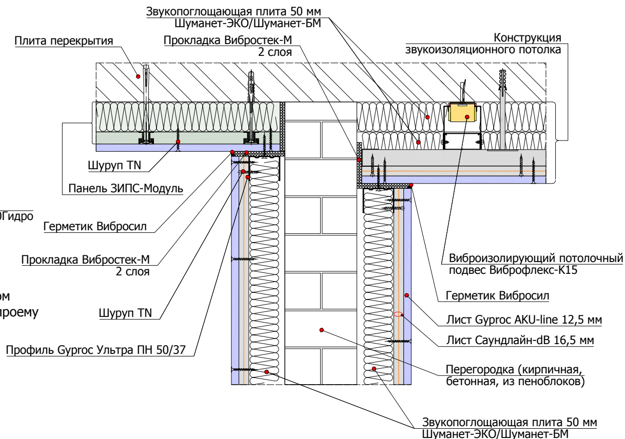
4.1.2 Примыкание облицовки стены на независимом каркасе 50 мм к панелям ЗИПС на потолочном перекрытии и подвесному звукоизолирующему потолку
