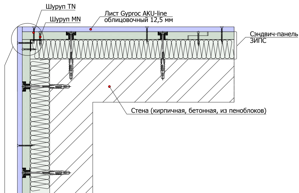
2.1.5 Узлы крепления панелей ЗИПС при монтаже внешнего угла
