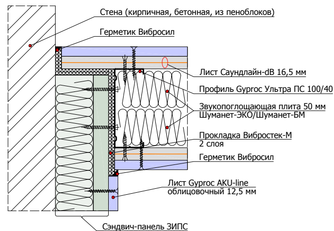
1.6.2 Угловое примыкание перегородки на одинарном каркасе 100 мм к панелям ЗИПС на стене
