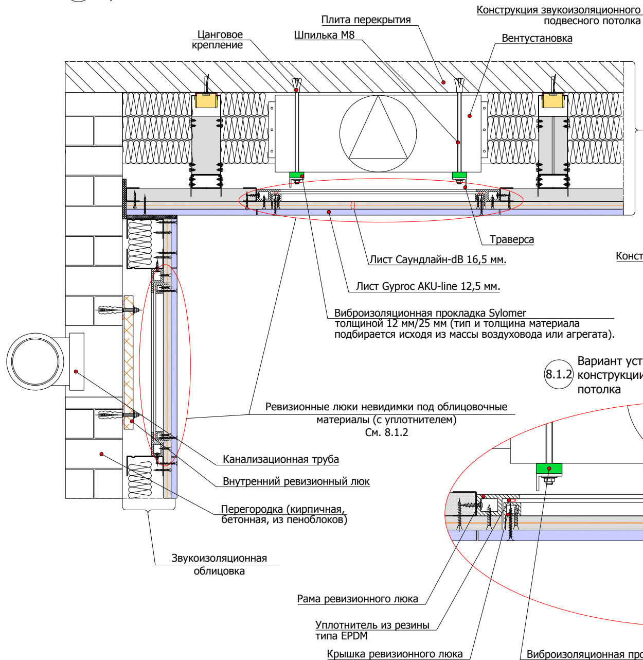
8.1.1 Схема устройства ревизионных люков в конструкциях звукоизоляционных потолков и облицовок
