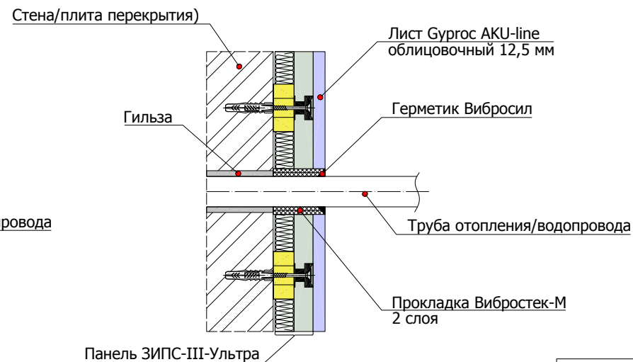
8.4.4 Схема пропуска труб отопления/водопровода через конструкцию панельной системы ЗИПС-III-Ультра
