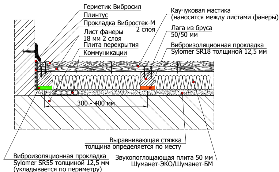
6.7.3 Схема примыкания конструкции пола по деревянным лагам с применением виброизоляционного материала Sylomer к стене и трубе отопления/водопровода (монтаж на ровное перекрытие)
