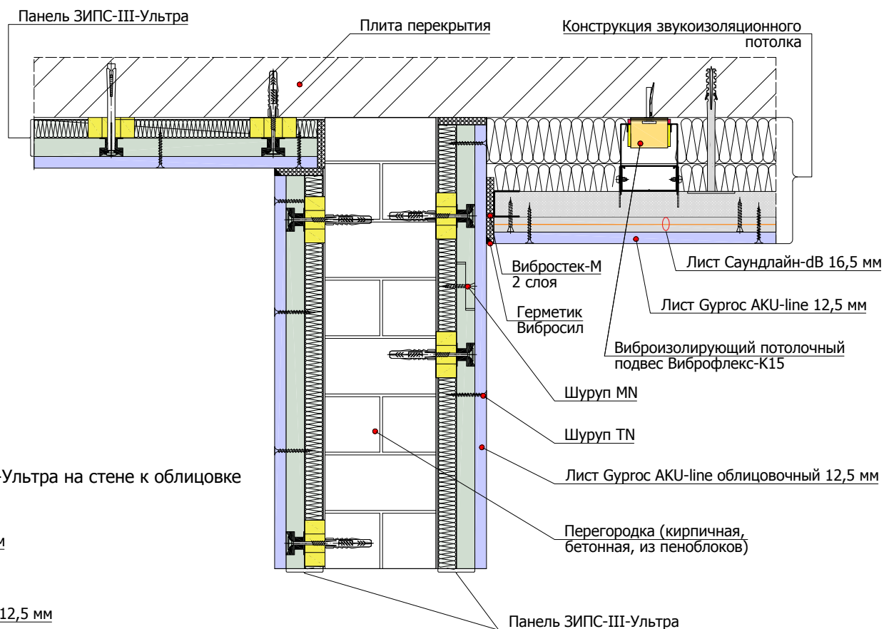
2.5.2 Примыкание панелей ЗИПС-III-Ультра к панелям ЗИПС-III-Ультра на потолочном перекрытии и подвесному звукоизолирующему потолку
