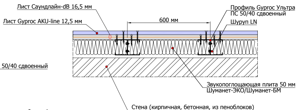
4.2.4 Облицовка стены на независимом сдвоенном каркасе 50 мм горизонтальный разрез
