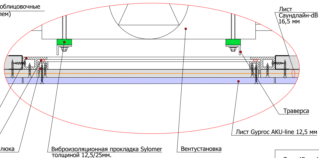
8.1.2 Вариант устройства ревизионного люка в конструкции звукоизоляционного подвесного потолка
