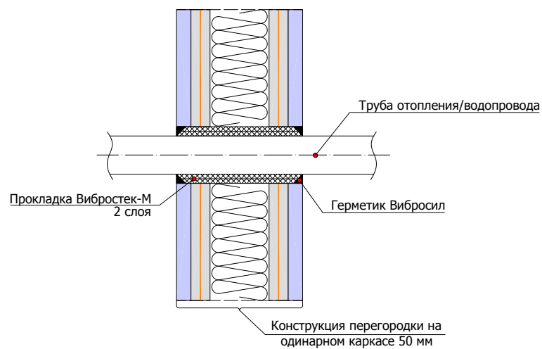
8.3.1 Схема пропуска труб отопления/водопровода через конструкцию перегородки на одинарном каркасе 50 мм
