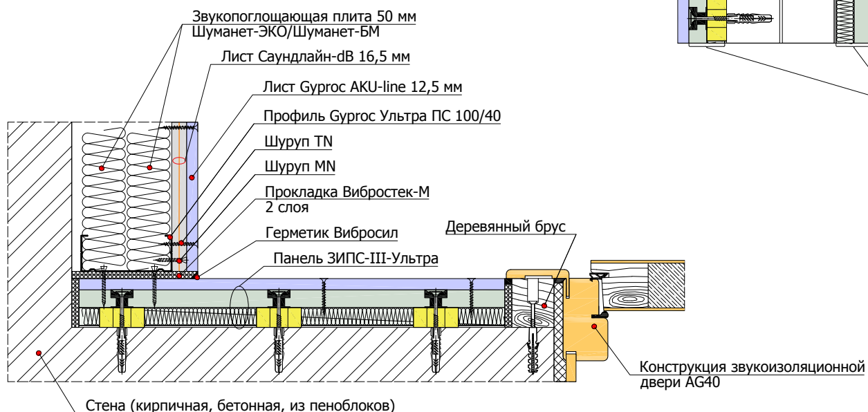
2.5.3 Угловое примыкание панелей ЗИПС-III-Ультра на стене к облицовке на каркасе 100 мм и дверному проему
