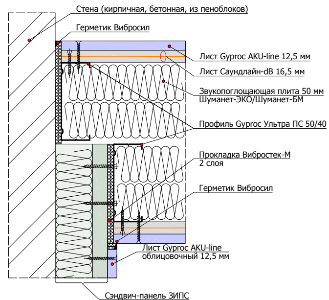
1.6.4 Угловое примыкание перегородки на двойном 2х100 мм (независимом) каркасе к панелям ЗИПС на стене
