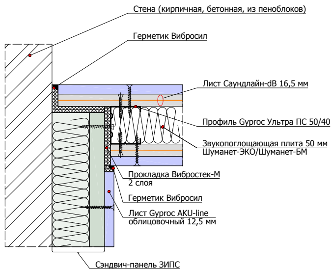
1.6.1 Угловое примыкание перегородки на одинарном каркасе 50 мм к панелям ЗИПС на стене
