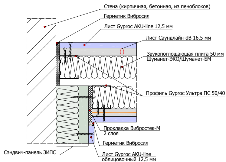
1.6.3 Угловое примыкание перегородки на двойном 2х50 мм (независимом) каркасе к панелям ЗИПС на стене
