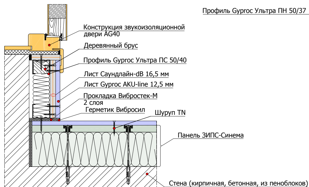
4.1.3 Угловое примыкание облицовки стены на независимом каркасе 50 мм к панелям ЗИПС на стене и дверному проему
