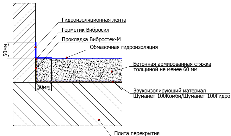
6.8.1 Схема устройства гидроизоляции в конструкции плавающего пола с применением звукоизолирующего материала Шуманет-100Комби/Шуманет-100Гидро
