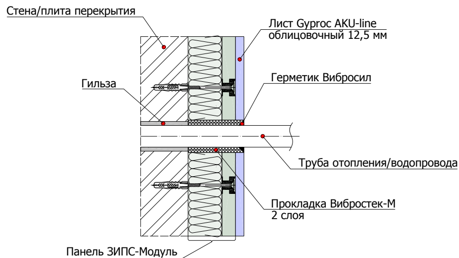
8.4.2 Схема пропуска труб отопления/водопровода через конструкцию панельной системы ЗИПС-Модуль
