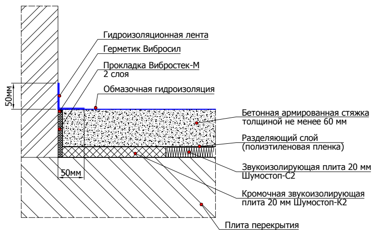
6.8.3 Схема устройства гидроизоляции в конструкции плавающего пола с применением звукоизолирующих плит Шумостоп в один слой
