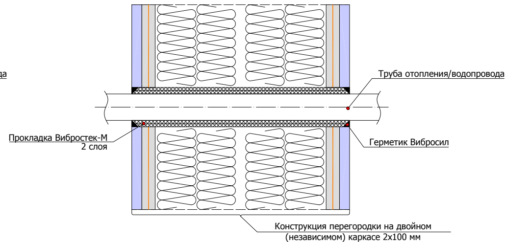
8.3.4 Схема пропуска труб отопления/водопровода через конструкцию перегородки на двойном (независимом) каркасе 2x100 мм
