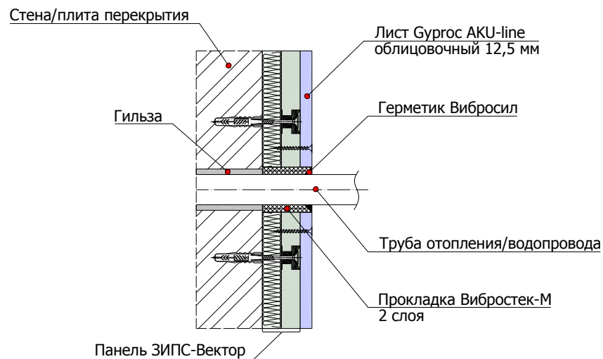
8.4.1 Схема пропуска труб отопления/водопровода через конструкцию панельной системы ЗИПС-Вектор
